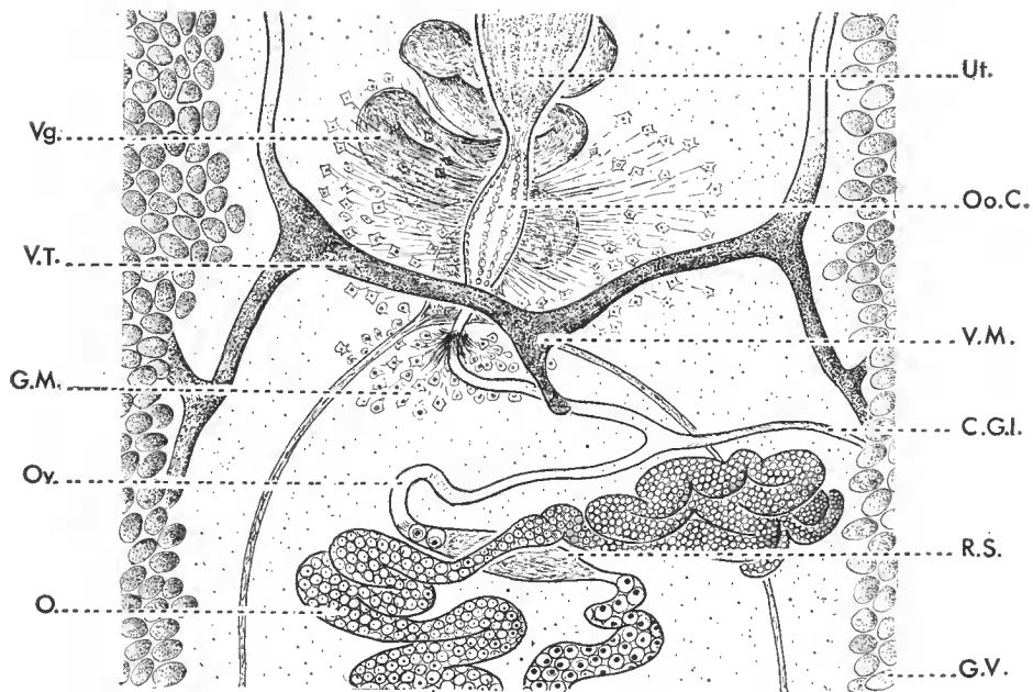
FIG. 3. — Détail de l'anatomie du genre Protocotyle n. g. C.G.I., canal génito-intestinal; G.M., glandes de Mehlis; G.V., glandes vitellogènes; O., ovaire; Oo.C., ootype côtelé; Ov., oviducte; R.S., réceptacle séminal; Ut., utérus; Vg., vagin; V.M., vitelloducte médian; V.T., vitelloducte transverse.
